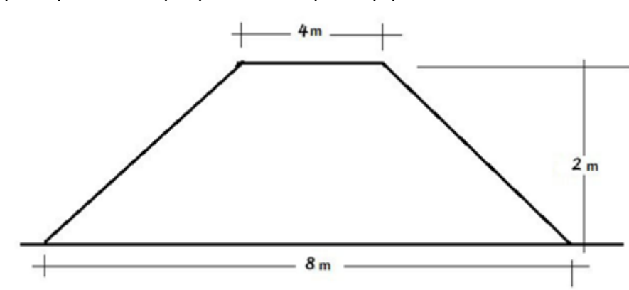
Διατομή Αργιλικού Αναχώματος μετά την επισκευή του.
