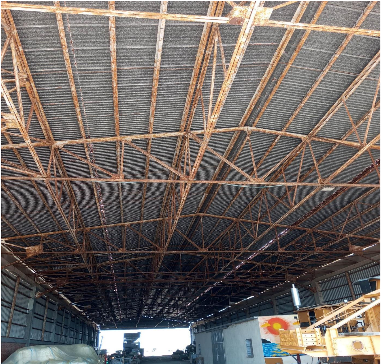
Άποψη του Υπόστεγου Οχημάτων (Εικ. 2)
